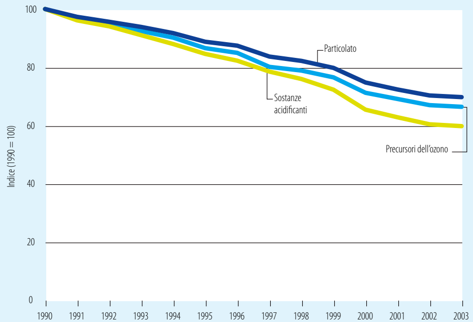
Grafico 3.1 — Evoluzione delle emissioni di inquinanti atmosferici prodotte dai trasporti, 1990-2003
