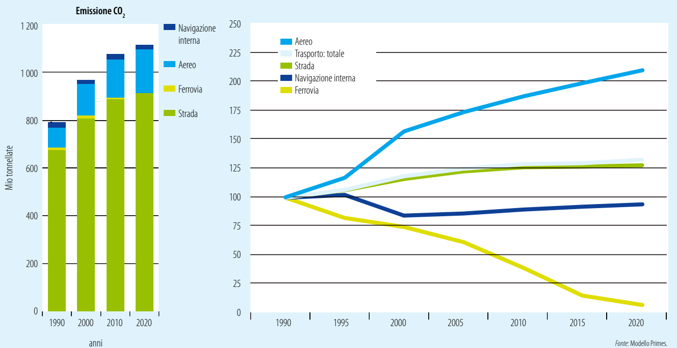
Grafico 3.2 — Evoluzione prevista delle emissioni di CO 2 prodotte dai trasporti ripartite per modo di trasporto (1990 = 100)
