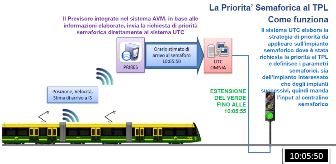
Figura 5-36 Schema di funzionamento priorità semaforica al TPL
