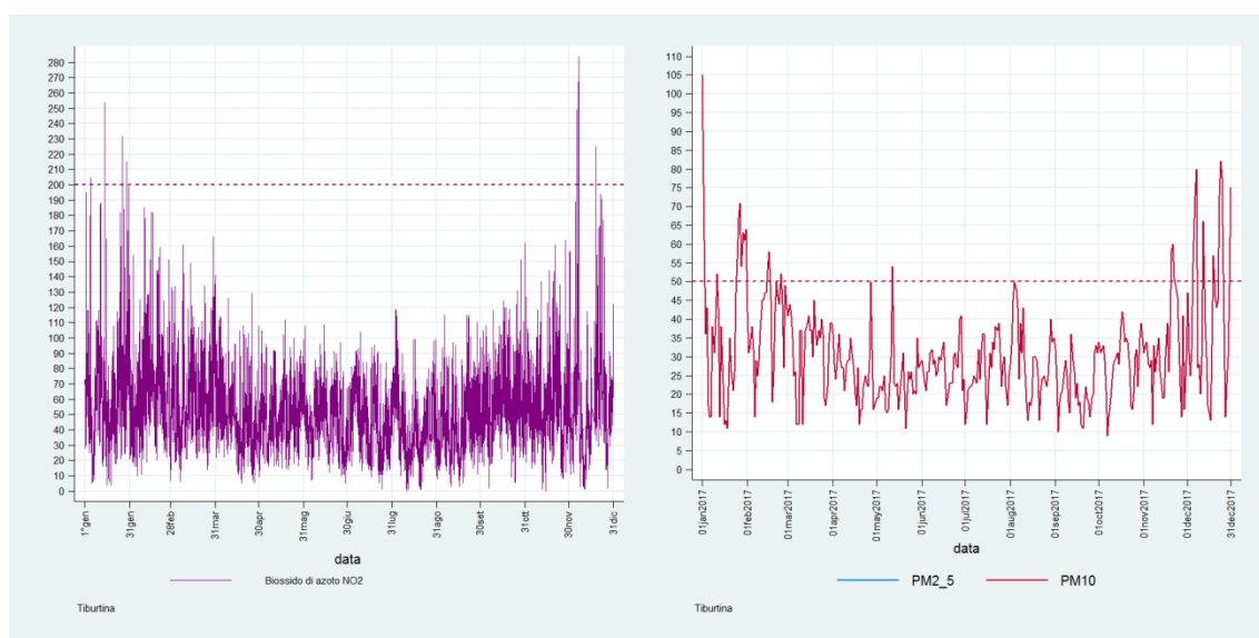
Figura 1-145 Concentrazioni di NO 2 (orarie) e PM 2.5 -PM 10 (giornaliere) nel 2017 (Fonte: ARPA Lazio) – Sezione di TIBURTINA
