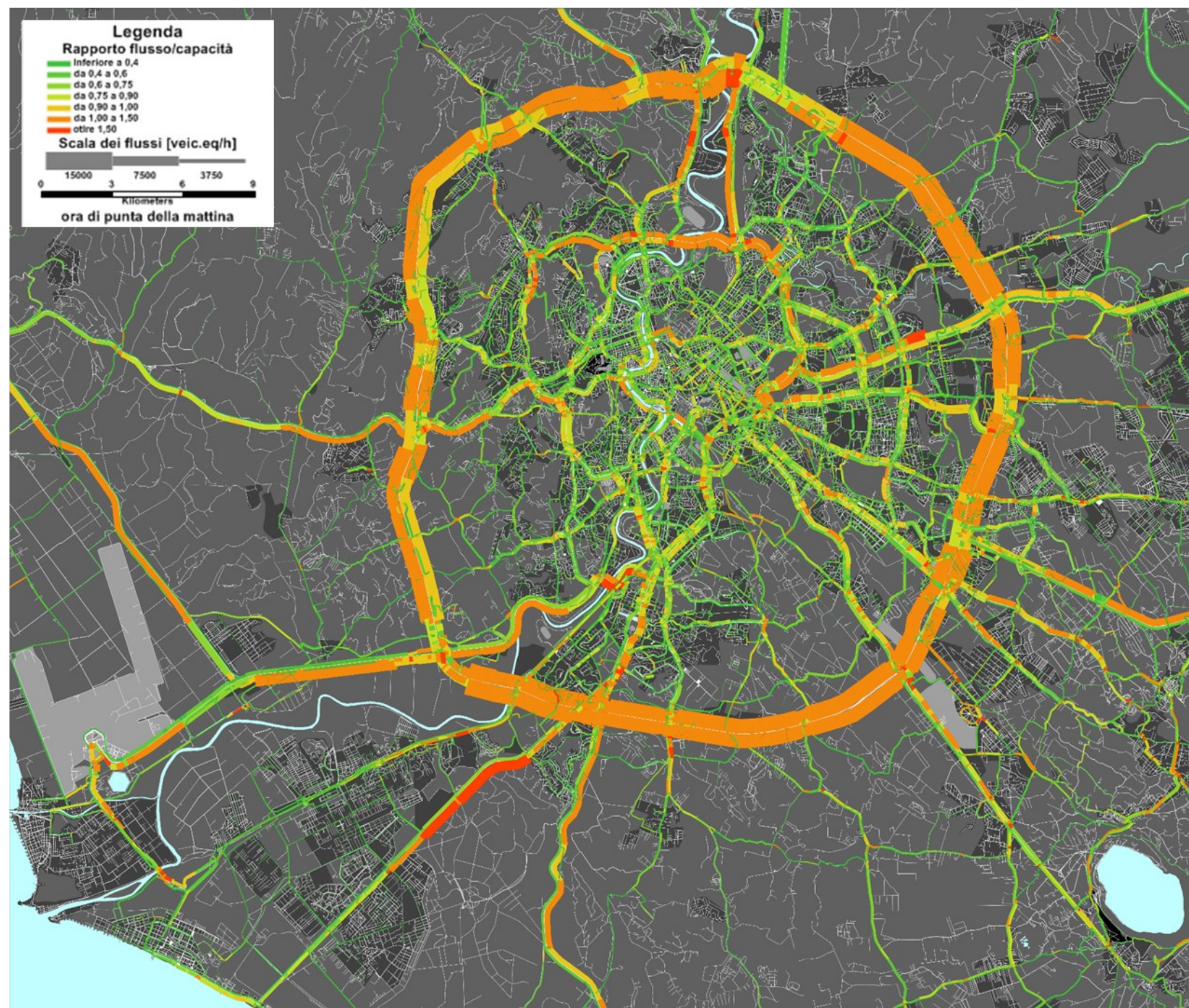
Figura 1-128 Assegnazione del sistema di trasporto privato ora di punta della mattina rapporto Flusso/Capacità – Scenario Attuale
