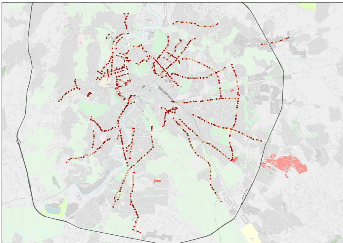
Figura 1-84 Distribuzione territoriale dei sistemi semaforici centralizzati
