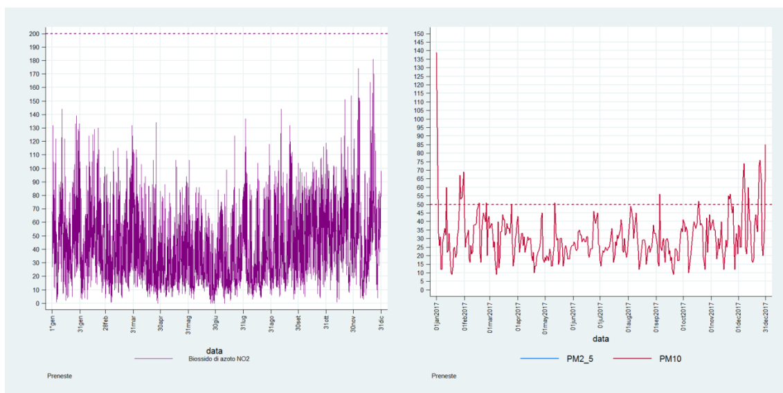
Figura 1-144 Concentrazioni di NO 2 (orarie) e PM 2.5 -PM 10 (giornaliere) nel 2017 (Fonte: ARPA Lazio) – Sezione di PRENESTE
